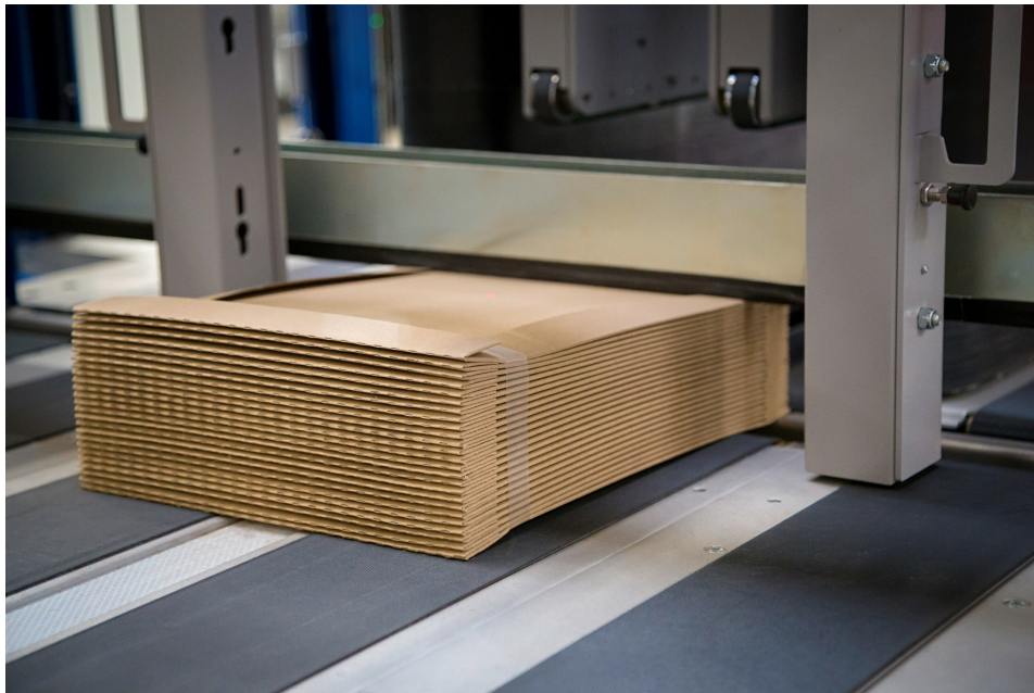
Ob Umreifen oder Banderolieren, die UCB bündelt Wellpappprodukte zuverlässig und gleichzeitig produktschonend. (© MOSCA)
