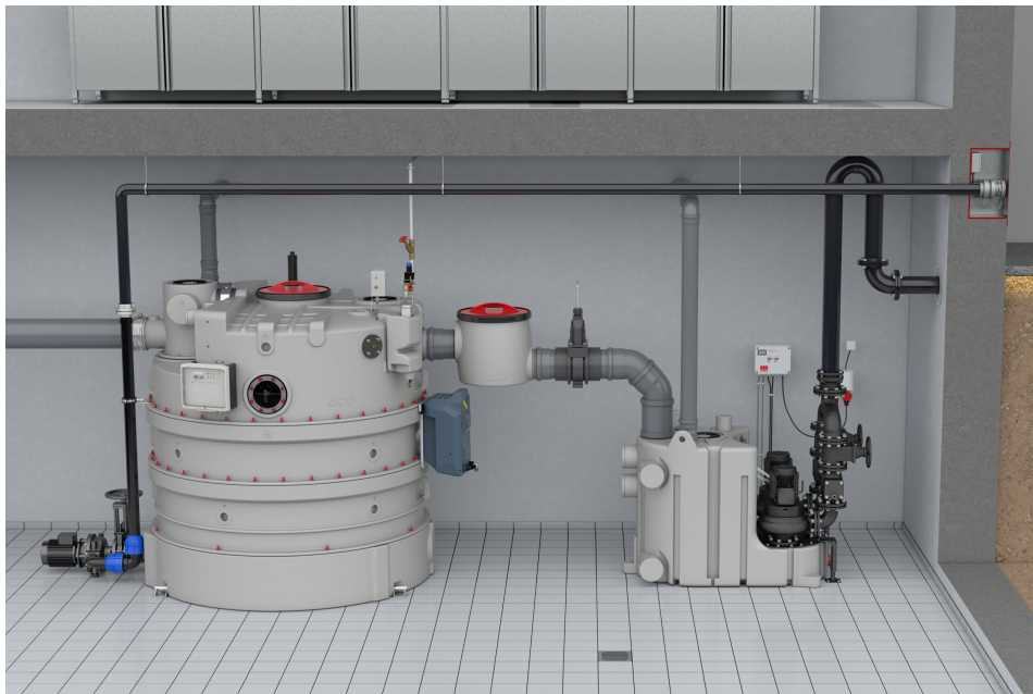
Einbaubeispiel: Entsorgungsleitung ohne Entsorgungspumpe. Bei Fettabscheidern ohne Entsorgungspumpen müssen Rohrmlenkungen und das finale Rohrstück vor dem Anschluss der Storz-Kupplung mit den regulären Sicherungsschellen aus dem Lieferprogramm fixiert werden. (©ACO)
